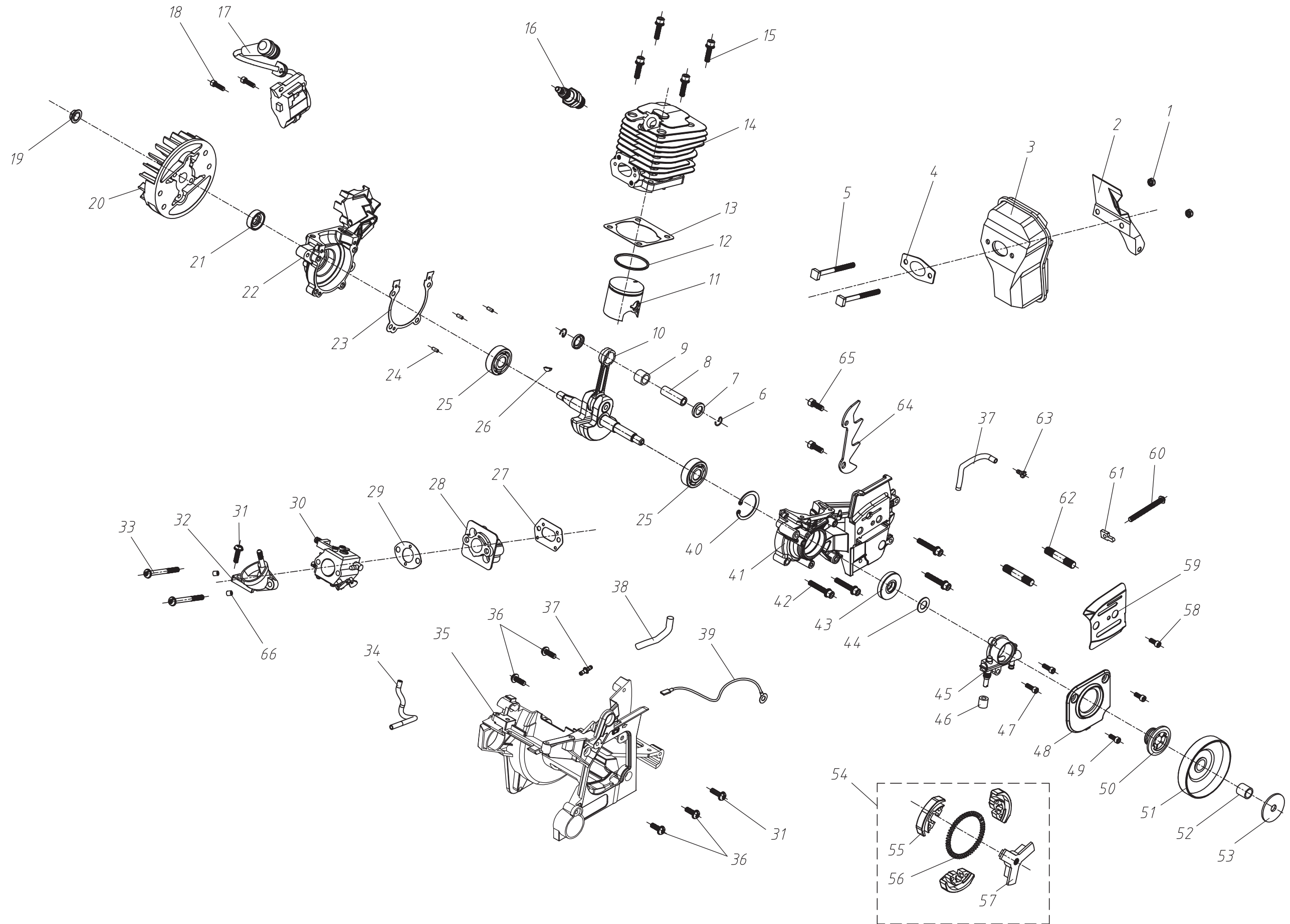
YD4 110油锯动力总成(普通)
